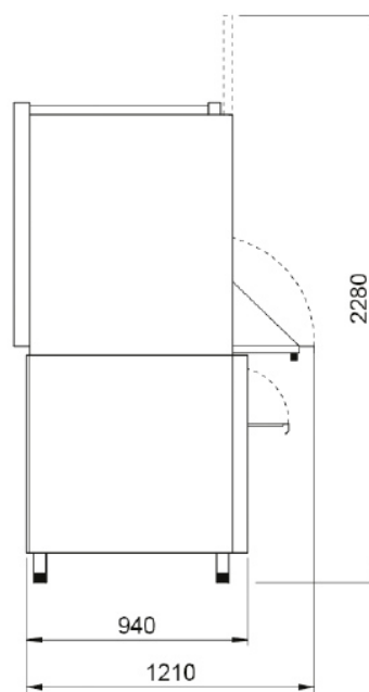
VISTA LATERAL
