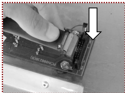
3- Conecte o terminal do chicote na placa NT.
