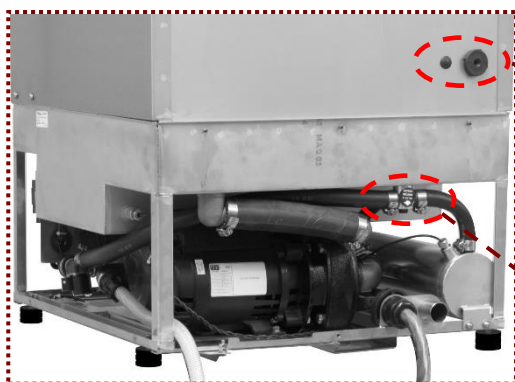
Ponto de entrada de secante
