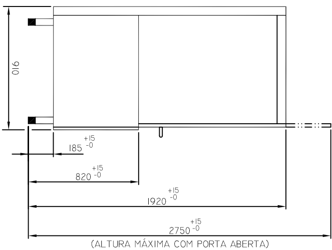
VISTA LATERAL
